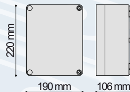
Размеры VK-25VCM
