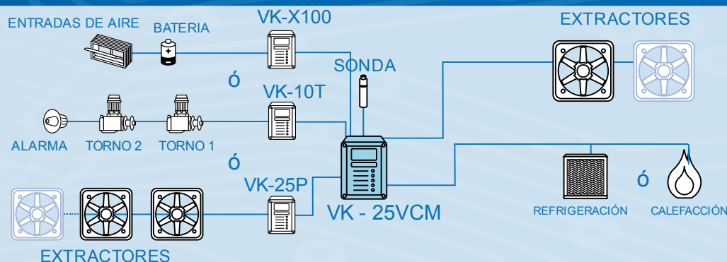
Esquema VK-25VCM
