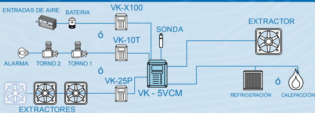
Esquema VK-5VCM
