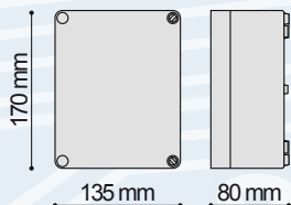
Dimensiones VK-5VCM
