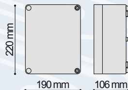
Dimensiones VK-25VCM
